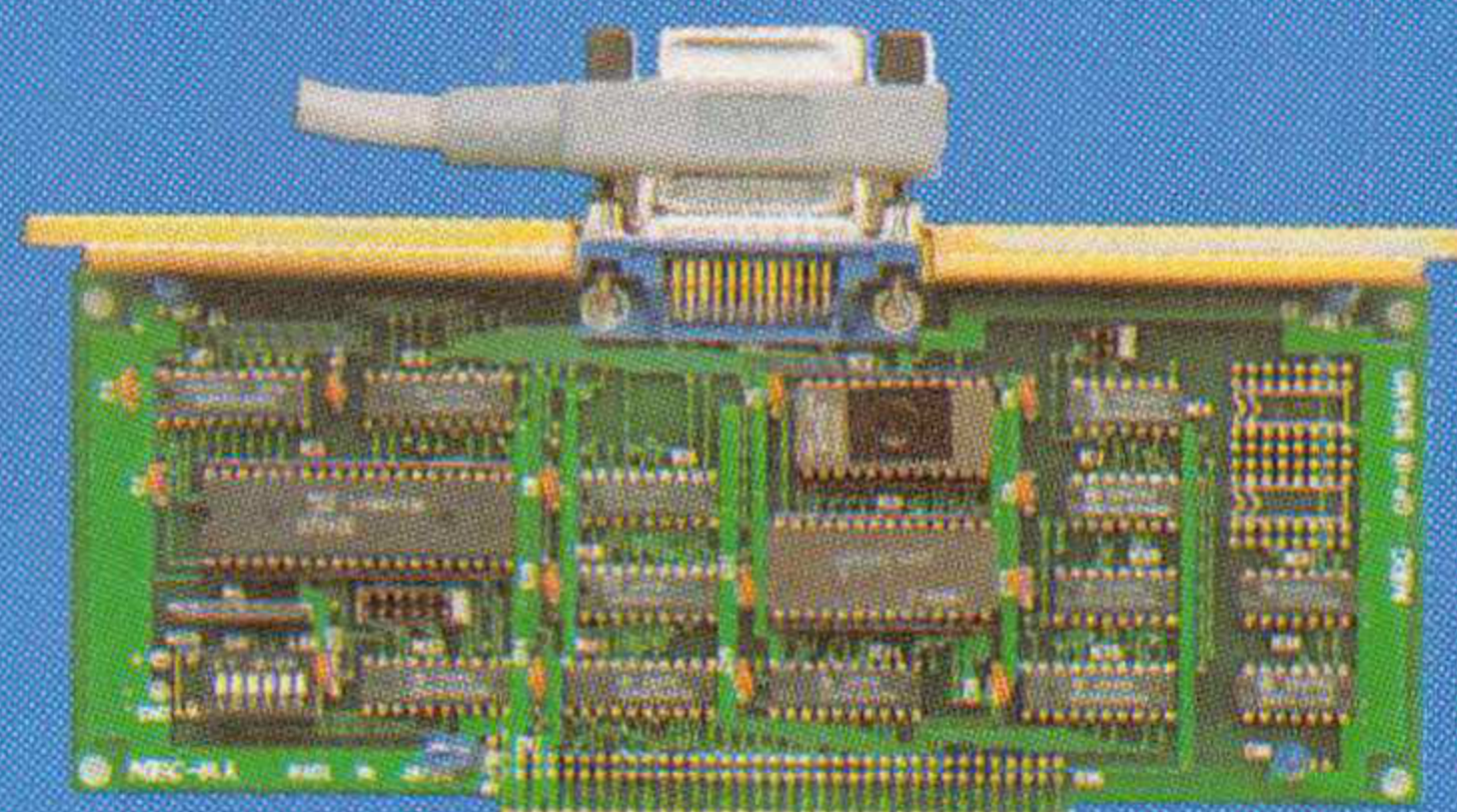
PC-8897 GP-IBインタフェースボード
