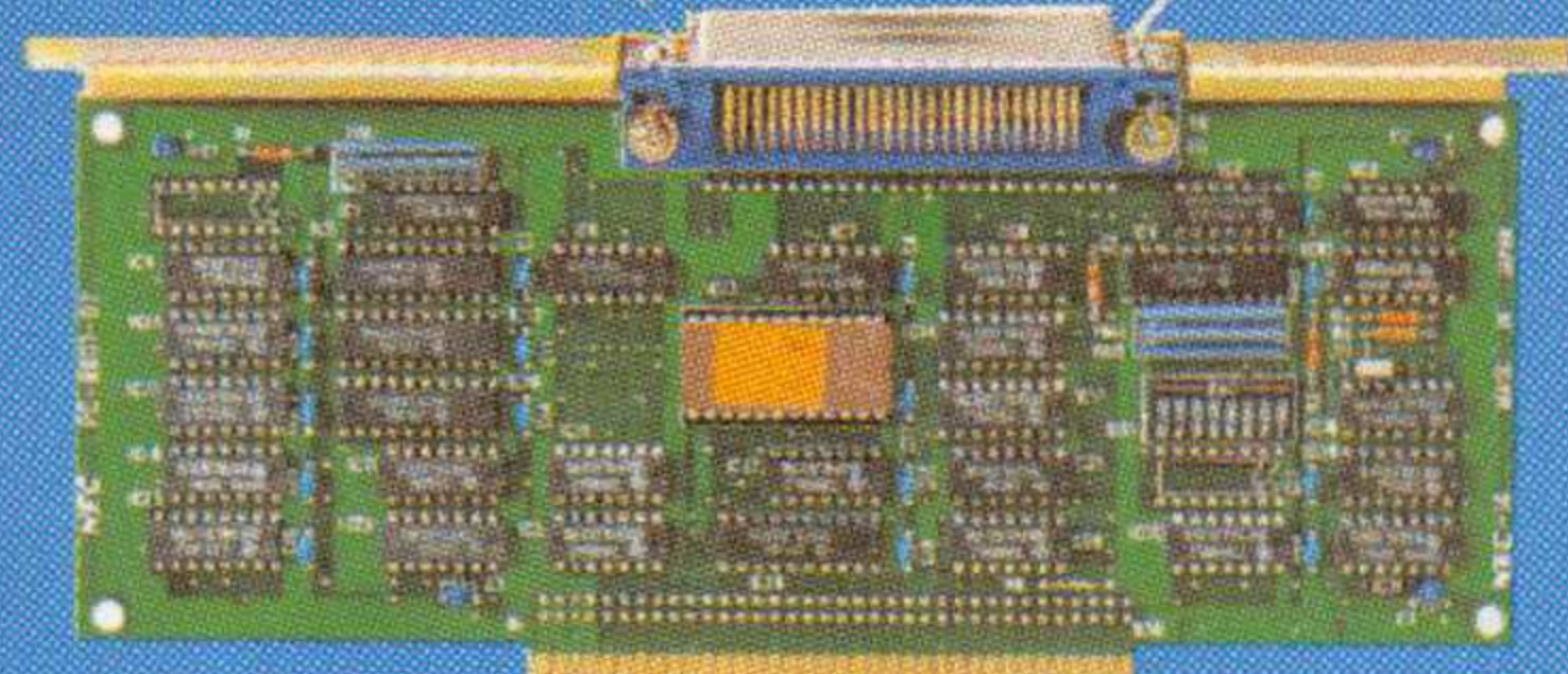
PC-8801-07 5インチ固定ディスク インタフェースボード
