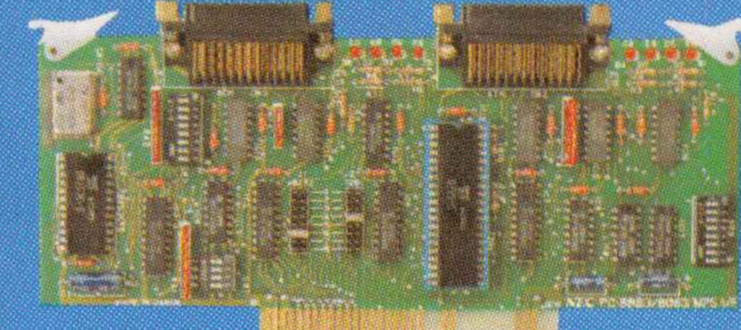
PC-8863 エミュレータ専用通信ボード
