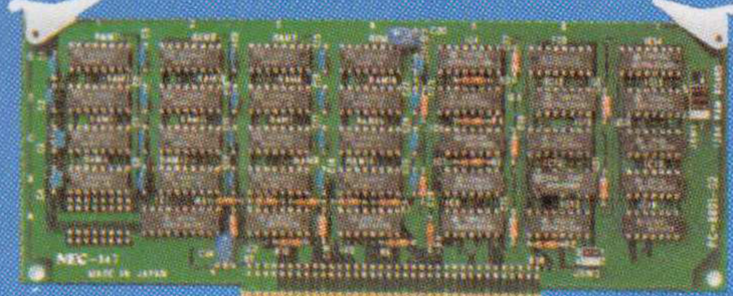
PC-8801-02N 増設RAMボード
